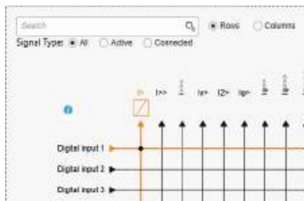
Figure 30 - DI input blocking connection
