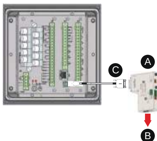
Figure 210 - VSE-001 module
