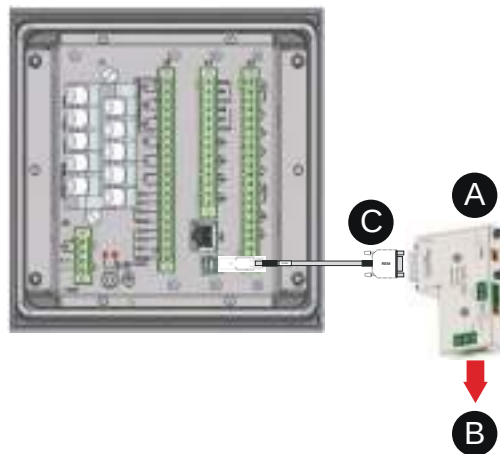
Figure 211 - VSE-002 module
